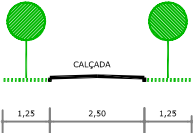
VIAS PARA PEDESTRES (V-7) PERFIL BÁSICO TRÁFEGO EXCLUSIVO DE PEDESTRES
