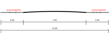
ESTRADAS MUNICIPAIS (V-5) PERFIL BÁSICO TRÁFEGO LOCAL
