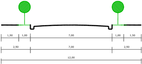
VIAS LOCAIS (V-4) PERFIL PARA VIAS DE ACESSO ÀS ESTRADAS NA ZONA RURAL TRÁFEGO LOCAL
