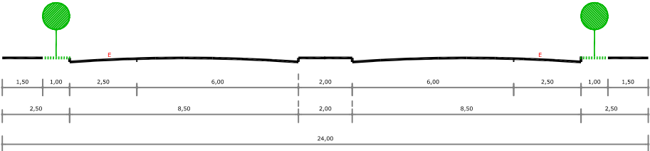
VIAS DE TRANSIÇÃO (V-1+V-6) PERFIL COM CANTEIRO CENTRAL EIXOS COMERCIAIS (AV. GAL. OSÓRIO E RUA DO COMÉRCIO)
