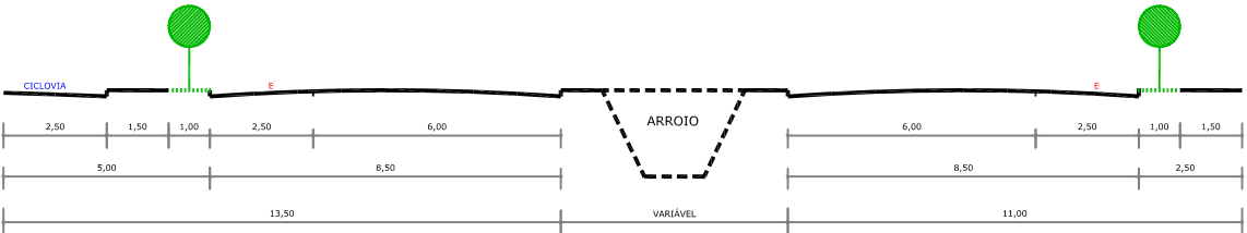
VIAS DE TRANSIÇÃO (V-1+V-6) PERFIL COM CICLOVIA ALTERNATIVAS PARA TRECHOS RODOVIÁRIOS URBANOS
