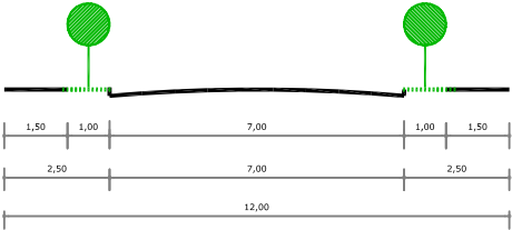
VIAS LOCAIS (V-4) PERFIL ALTERNATIVO TRÁFEGO LOCAL (LOTEAMENTOS FORA DA ÁREA URBANA)
