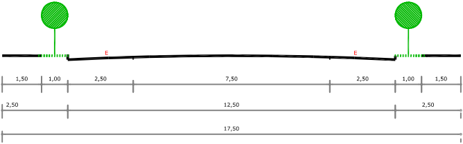
VIAS DE TRANSIÇÃO (V-1) PERFIL BÁSICO
