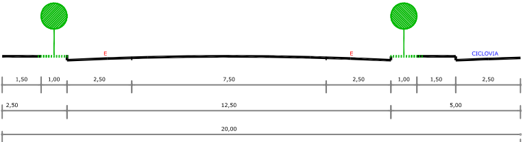
VIAS DE TRANSIÇÃO (V-1+V-6) PERFIL COM CICLOVIA
