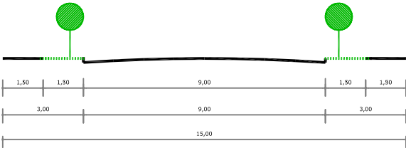
VIAS LOCAIS (V-4) PERFIL PARA VIAS DE ACESSO ÀS ESTRADAS NA ZONA RURAL TRÁFEGO LOCAL
