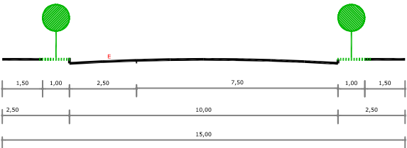
VIAS ARTERIAIS (V-2) PERFIL BÁSICO CONEXÕES INTRA-URBANAS (MUNDO NOVO)
